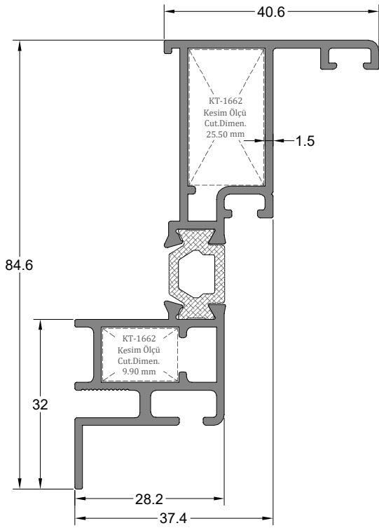
Tek Cam Yalıtımlı Kasa Profili THERMAL BREAK SINGLE GLAZING FRAME PROFILE
