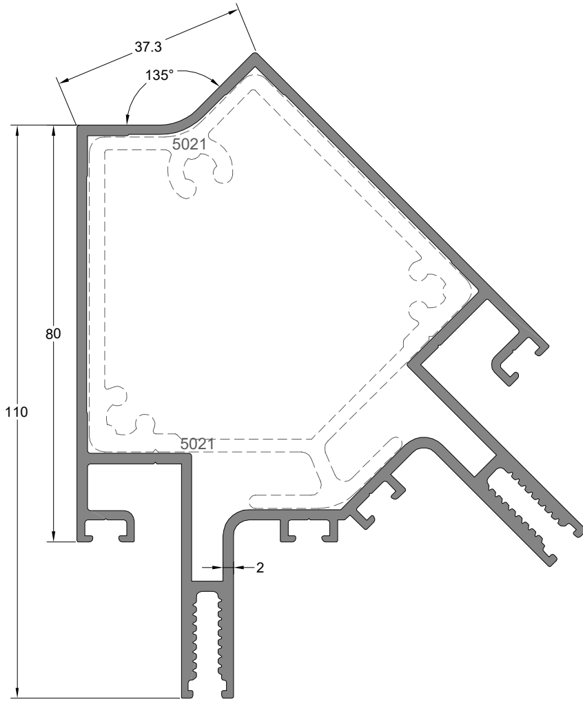
135° Köşe Dönüş Profili 135° CORNER PROFILE
