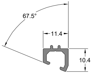
135° Köşe Dönüş Çita Profili 135° CORNER BEAD PROFILE
