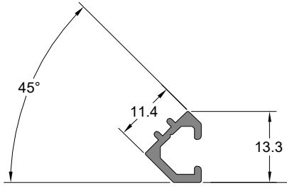
90° Dıştan Dönüş Çita Profili 90° CORNER BEAD PROFILE
