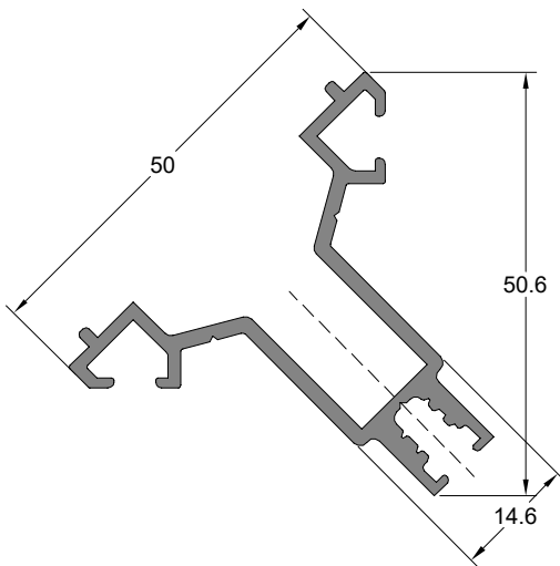
90° Dıştan Köşe Dönüş Adaptör Profili 90° CORNER COVER ADAPTER PROFILE
